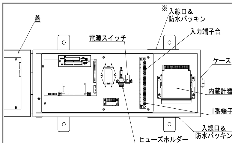
ケース内部
