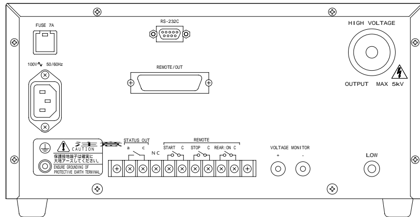
裏面図
