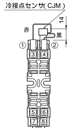
端子番号図 (単位: mm)
