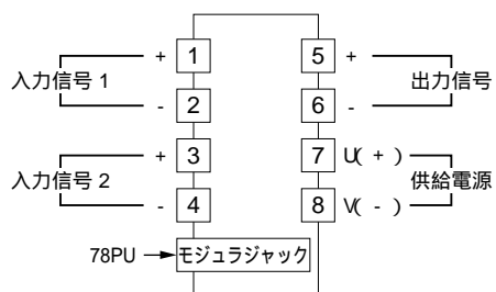
端子接続図
