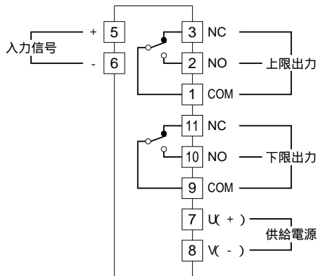
端子接続図
