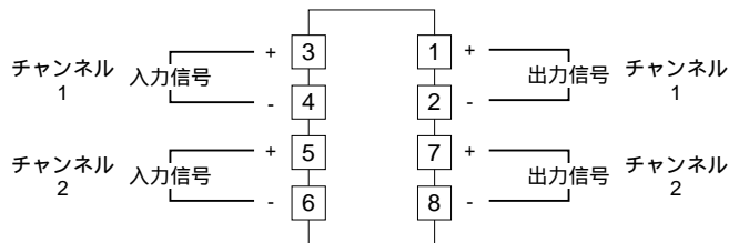
端子接続図
